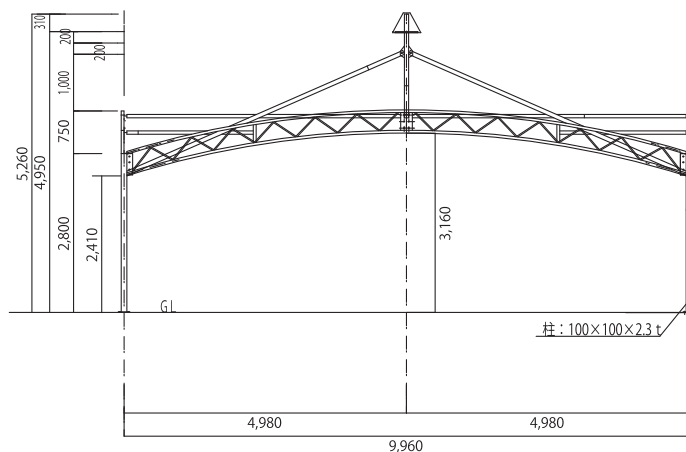
立面図 ①
