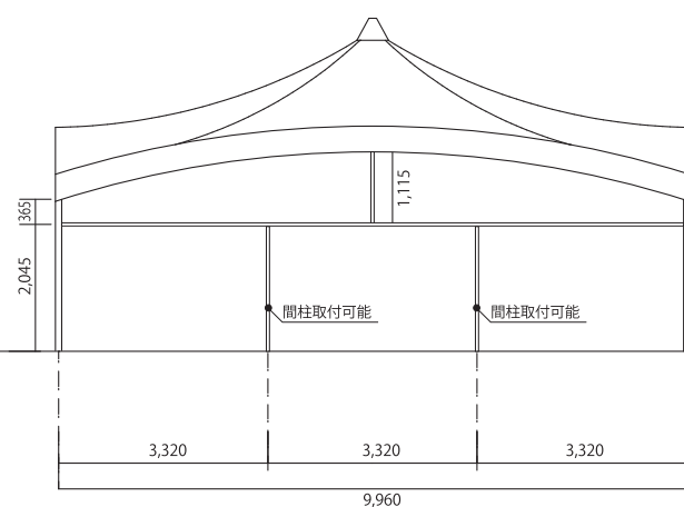
横幕: 半月幕用フレーム
