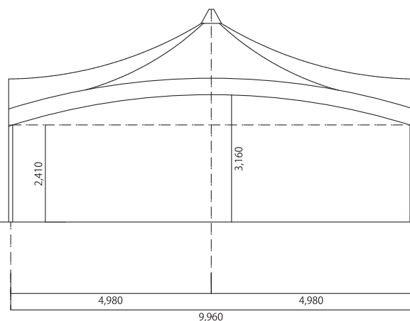
立面図 ②
