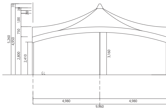
横幕: 1枚幕用フレーム
