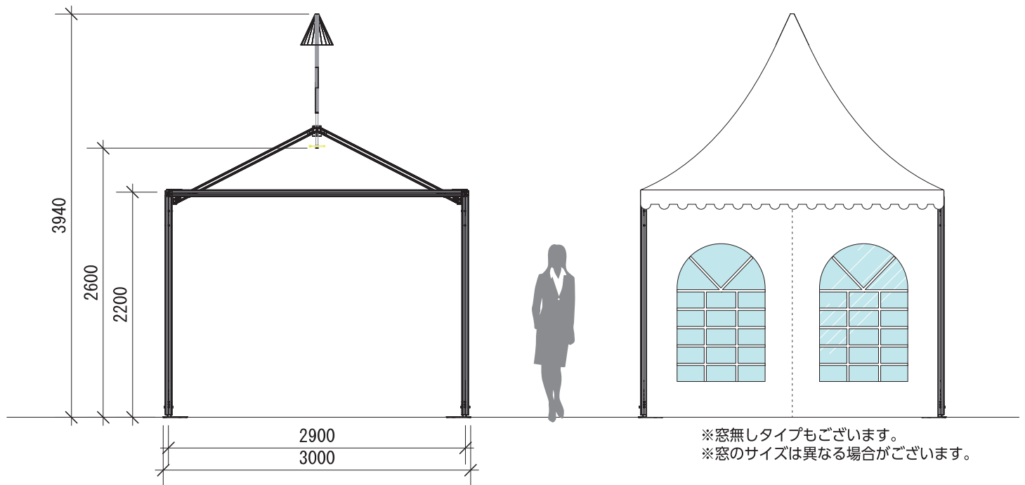
立面骨組図
