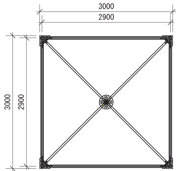
屋根伏骨組図
