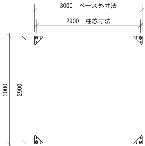
基礎ベース図
