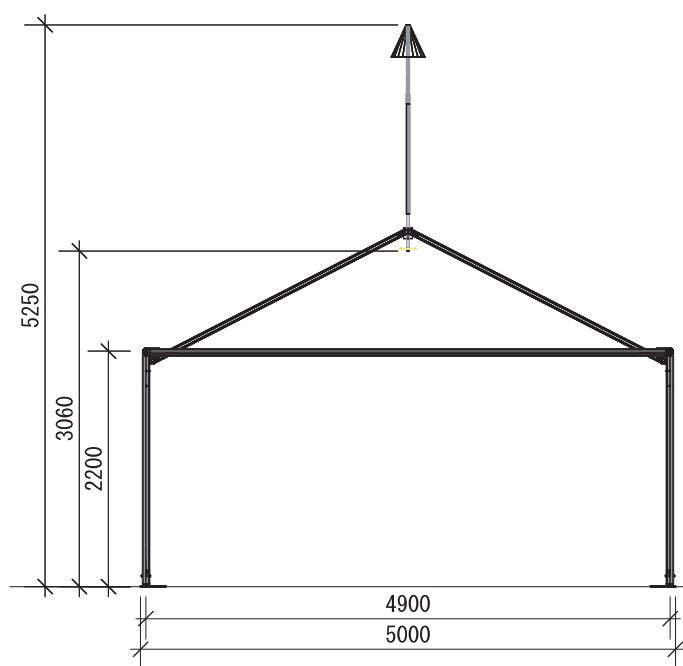
立面骨組図
