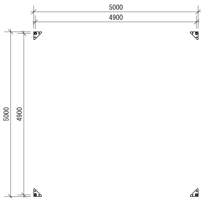
基礎ベース図
