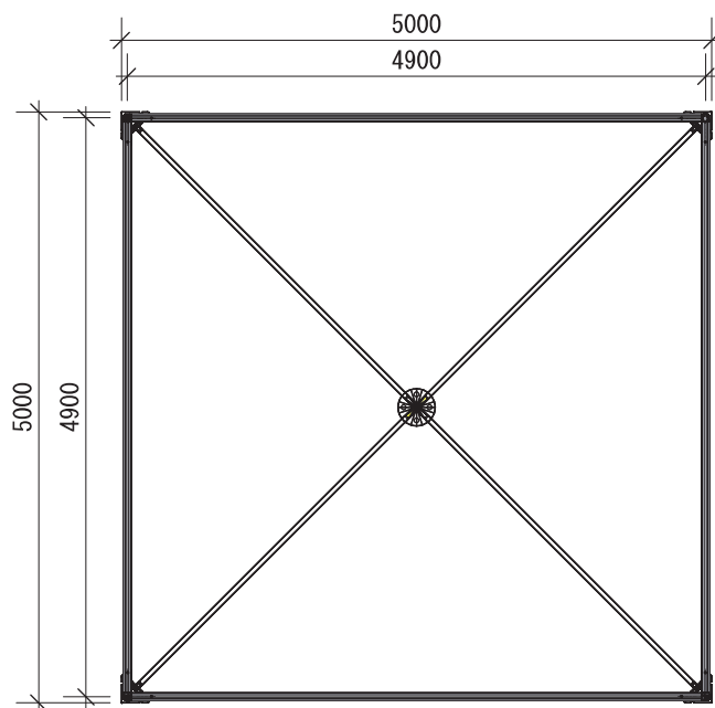
屋根伏骨組図
