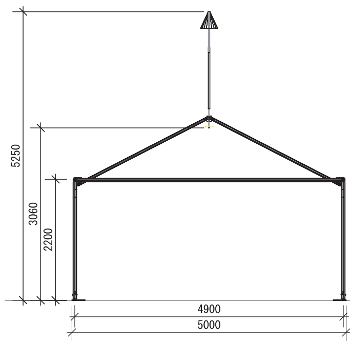
立面骨組図
