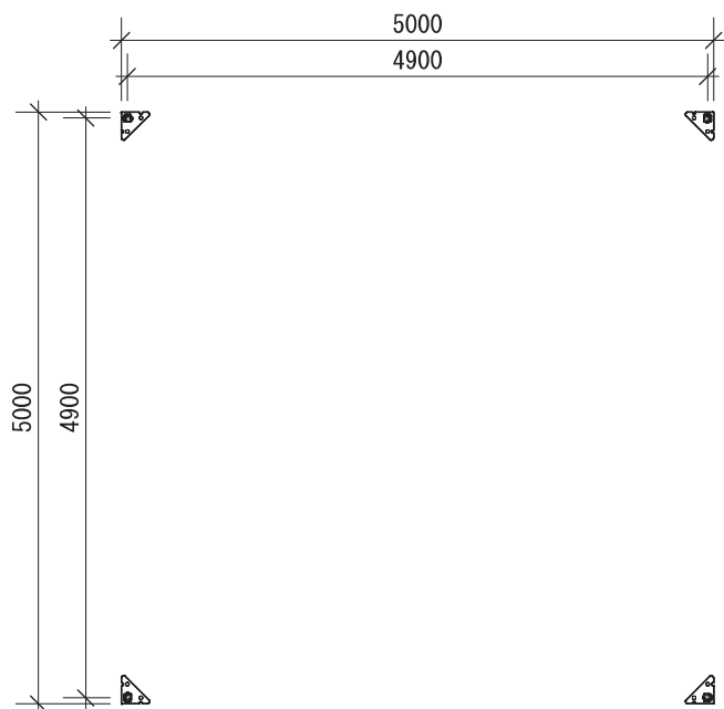
基礎ベース図
